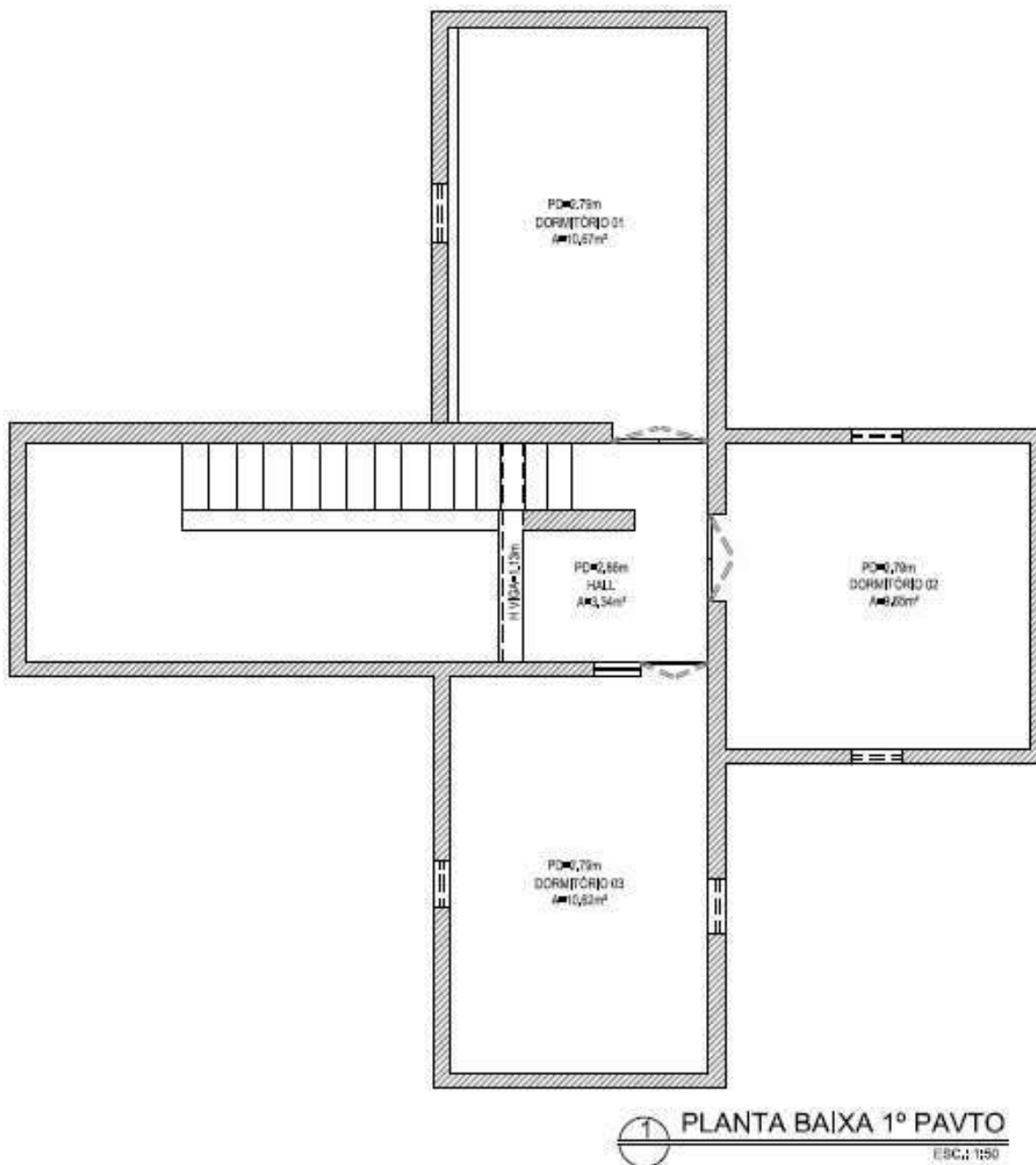
Figura 11: Planta baixa do Instituto Tembetá - IT.
