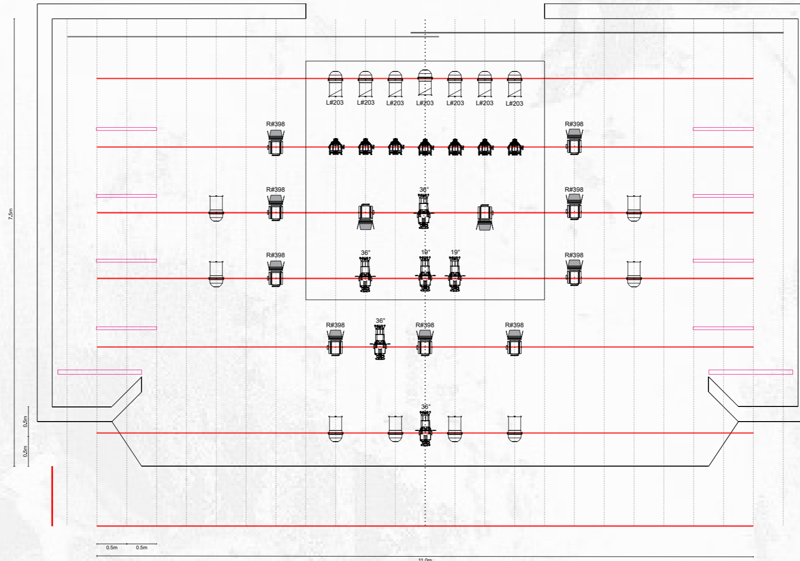
PLANTA DE VARAS_001
