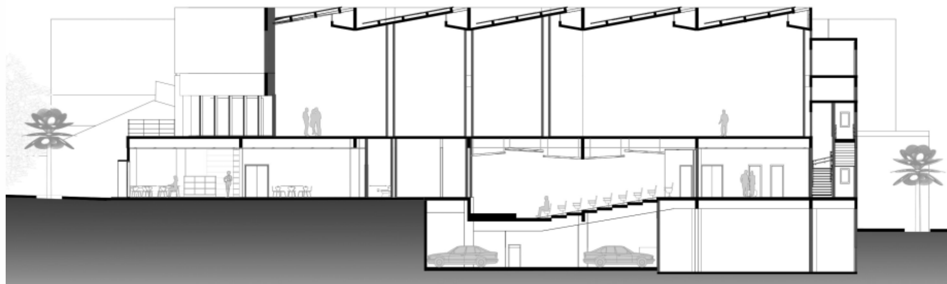
Corte B 0 1 5 15
